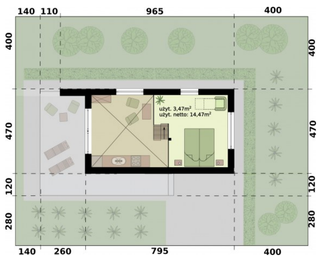
rzut parteru
