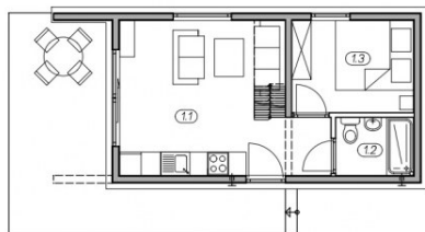
rzut parteru
