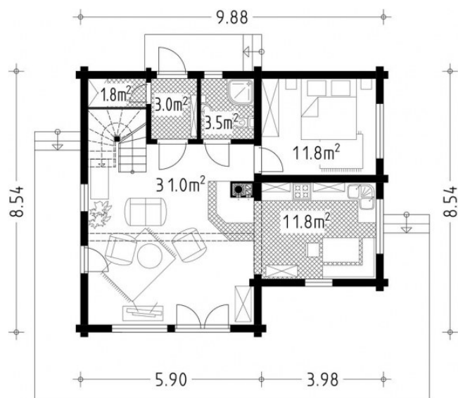
rzut parteru
