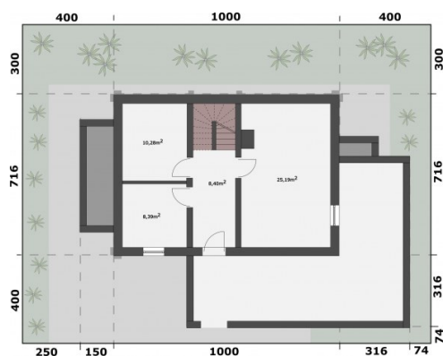
rzut piwnic
