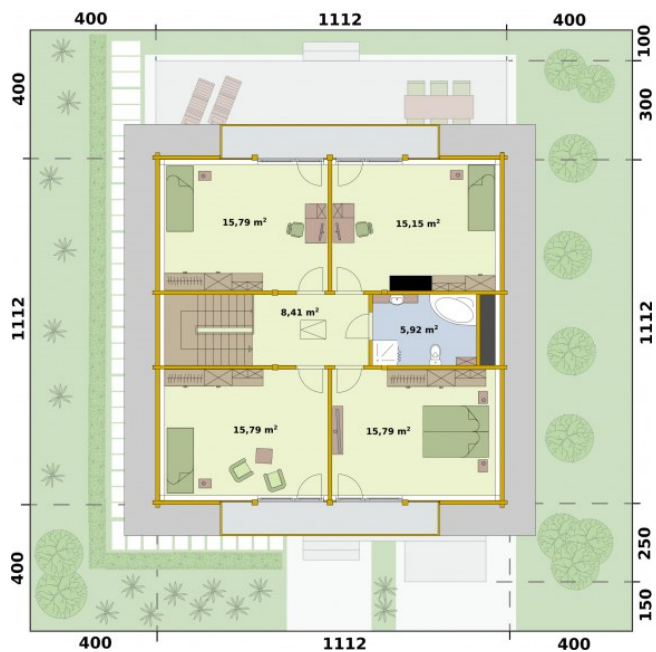
rzut poddasza
