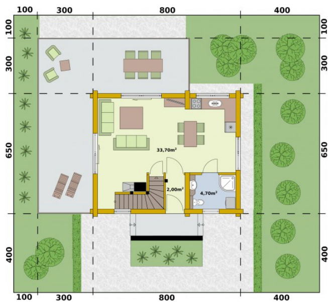
rzut parteru
